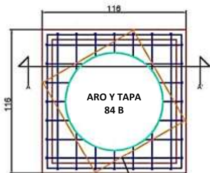
PLANTA TAPA VARILLA DE 1/2" DE Ø PARA REFUERZO DEL BROCAL F'y = 411970.3 KPa (4,200 Kg/cm 2 )
